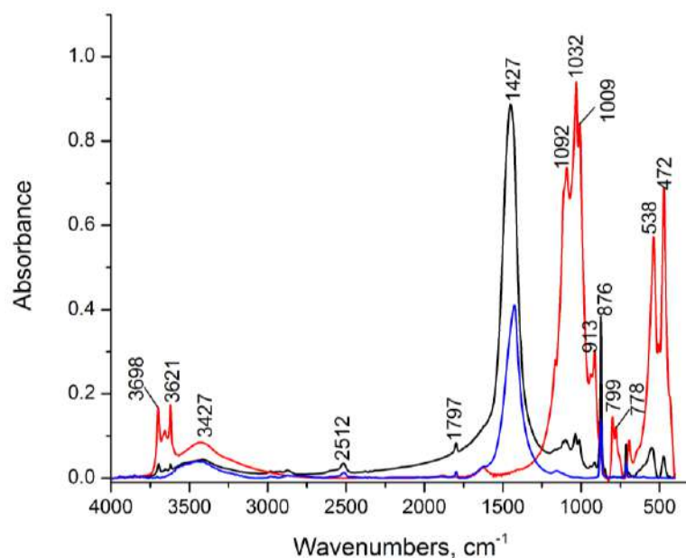
Абсорбционни ИЧ спектри (в таблетка KBr) на червената проба (в черно); референтен \text{CaCO}_3 (в синьо) и референтна червена охра (в червено)
