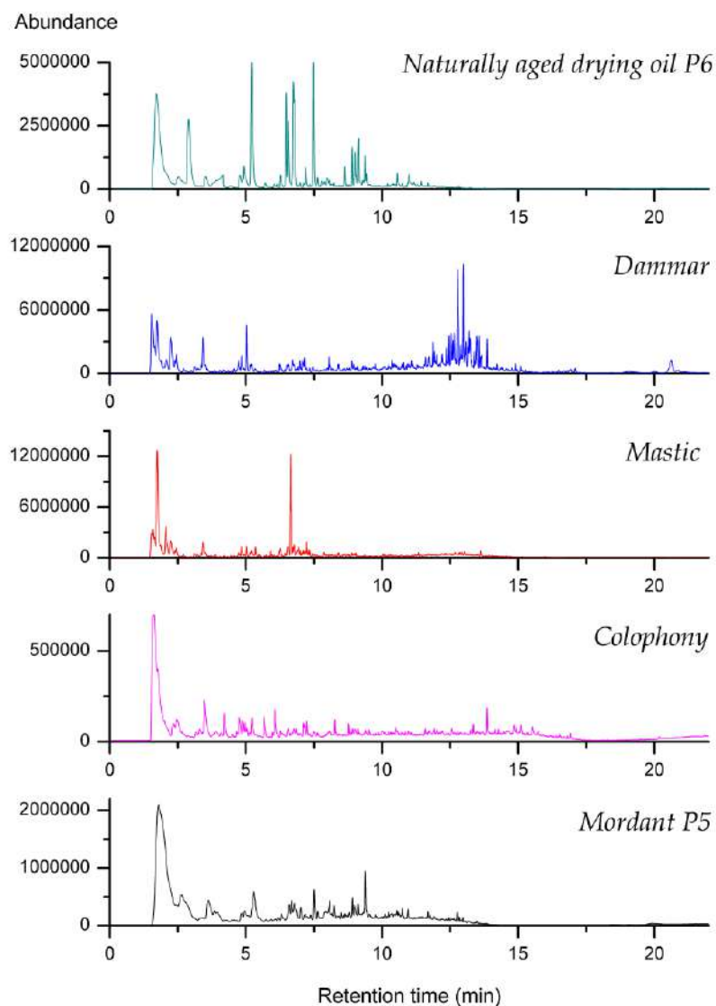
GC хроматограми на колофон, мастикс, дамара, миксиона за позлатата (P5) и естествено остаряло съхнещо масло (P6)
