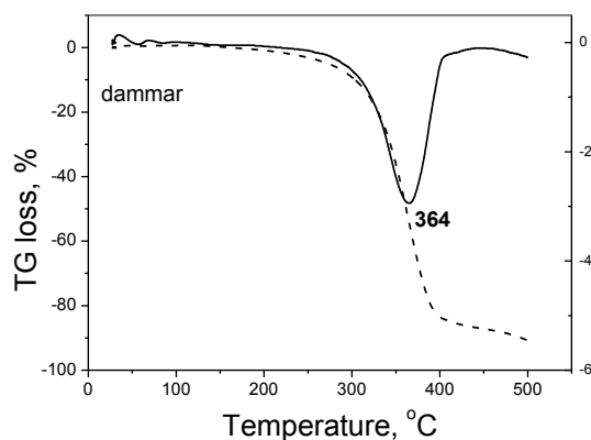
TGA анализ на растителна смола дамара
